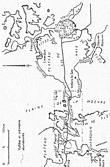
- La Moselle, l'Ingrès, la Moselle et la Meurthe dans la région comprise entre Void et Nancy.
