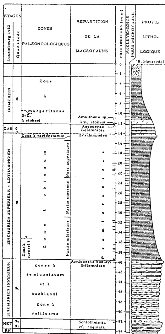
— Coupe stratigraphique du sondage de Laneuveville-devant-Nancy.
